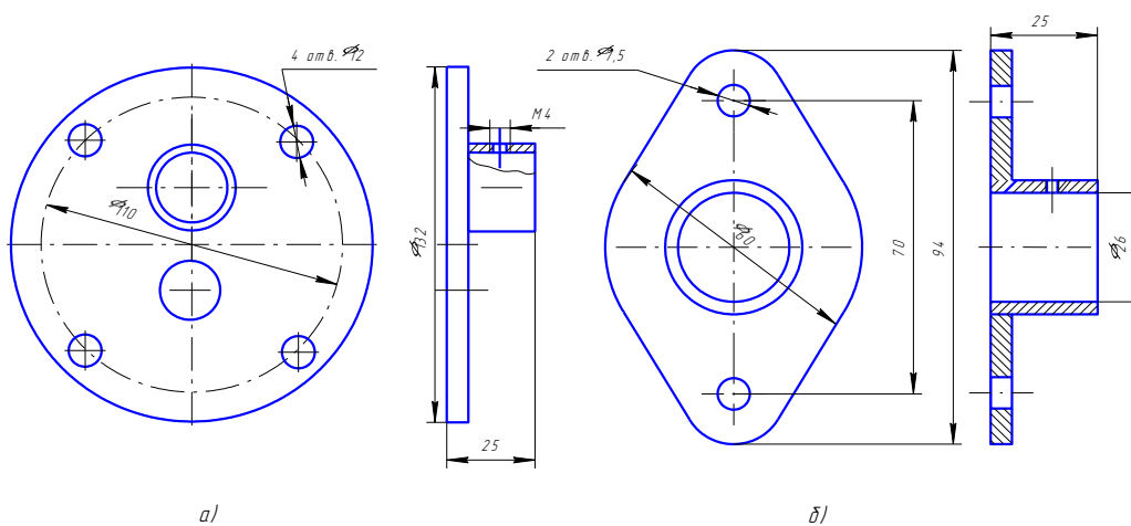
Рис.9. Фланцы
